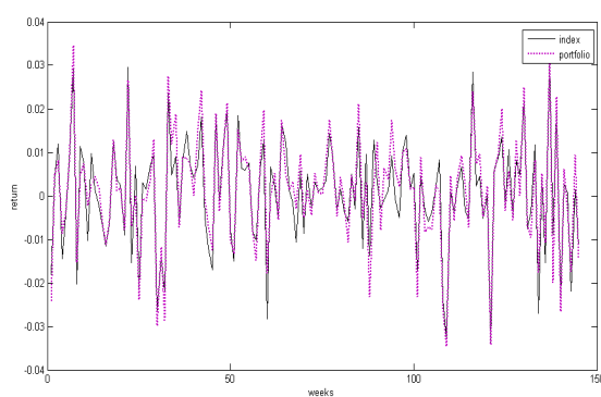
شکل ۱) ردیابی شاخص S&P500 با k=15 ، دوره آموزش
