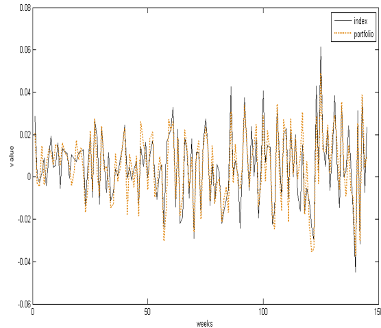
شکل ۲) ردیابی شاخص S&P500 با K=15 ، دوره سنجش
