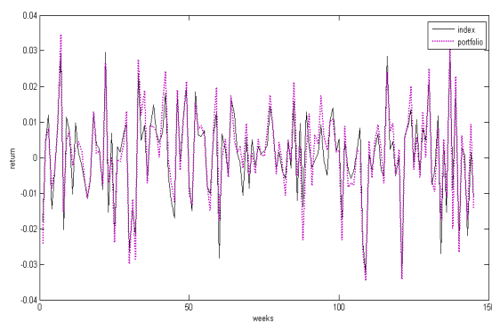
شکل ۱) ردیابی شاخص S&P500 با k=15 ، دوره آموزش
