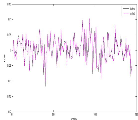
شکل ۳) ردیابی شاخص Hang Seng با k=5 ، آموزش
