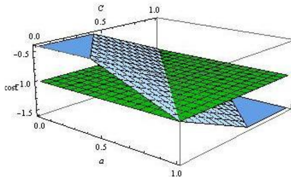
شکل ۳. هزینه گره‌ها وابسته به مقادیر c و k (محور x نشان‌دهنده a ، محور y نشان‌دهنده cost و محور z نشان‌دهنده C است).
