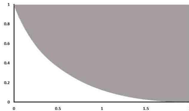
شکل ۲. مقدار فاکتور تخفیف زمانی که استراتژی آستانه تعادل نش است و به نسبت m/b بستگی دارد. محور عمودی نشان‌دهنده \delta و محور افقی نشاندهنده m/b است.
