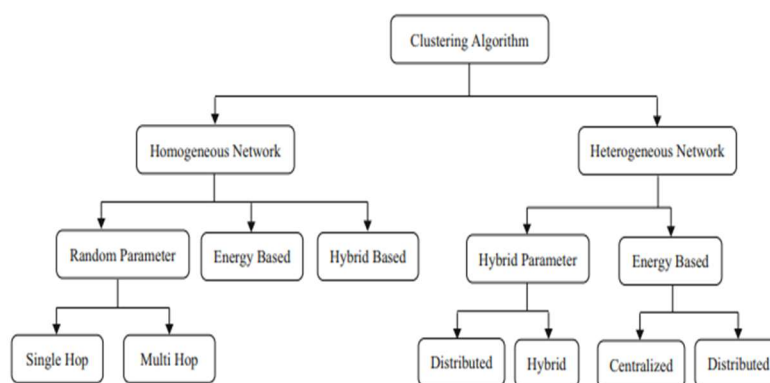
شکل ۱. دسته‌بندی الگوریتم‌های خوشه‌بندی
